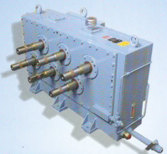
Rollenantriebe
