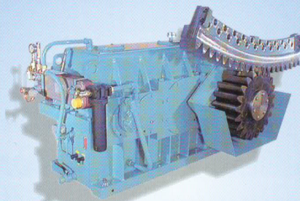
Trommelantriebe
