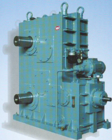
Pressengetriebe
